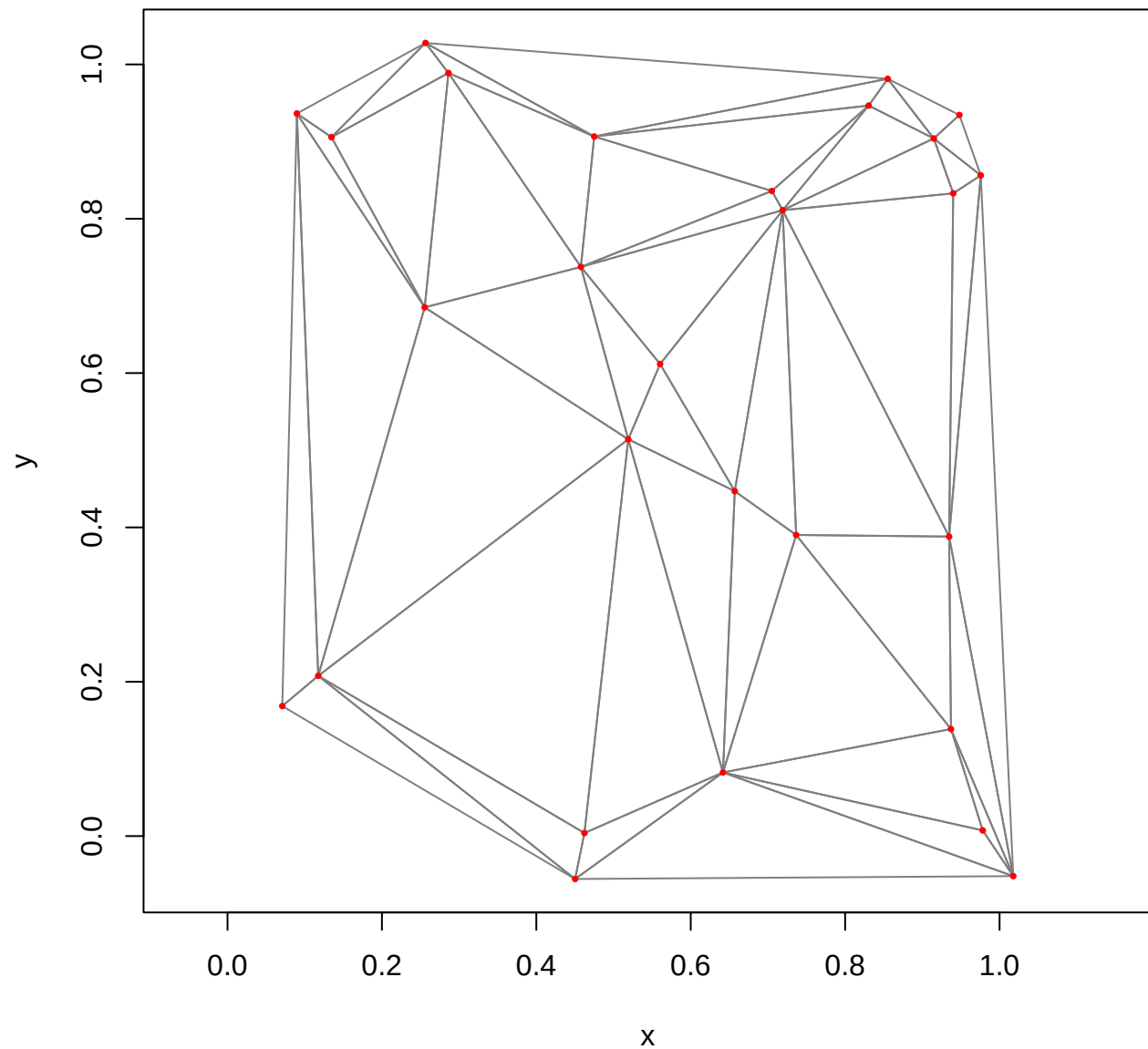
tulpa_mesh
