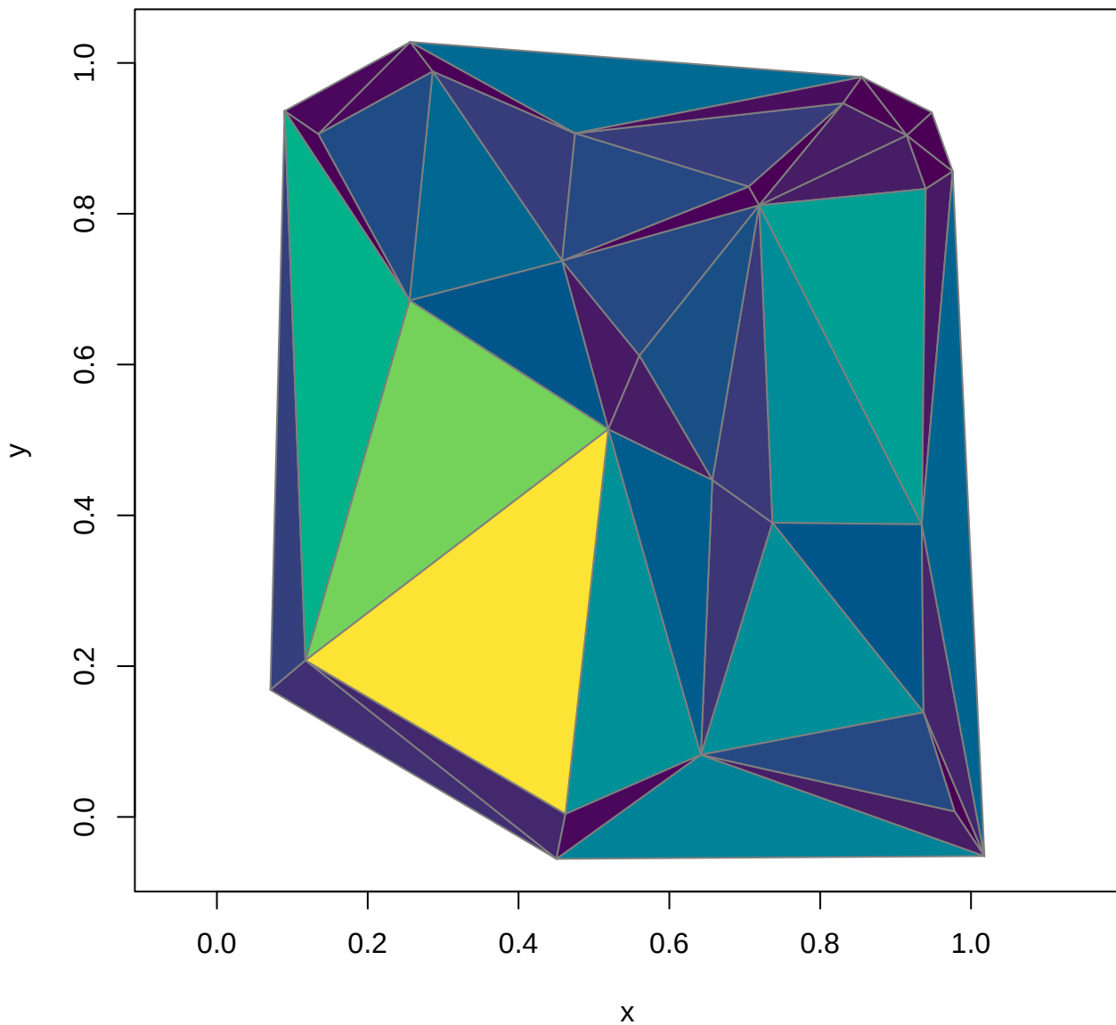
tulpa_mesh
