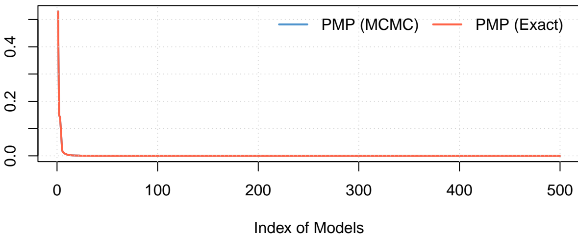
Posterior Model Probabilities (Corr: NA)
