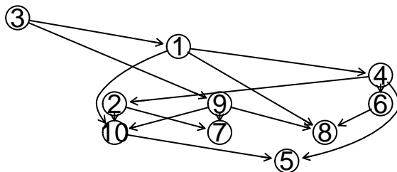
bipartite
