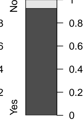
Node 9 (n = 274)
