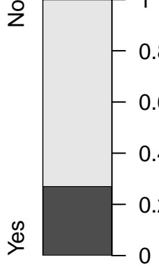
Node 5 (n = 48)
