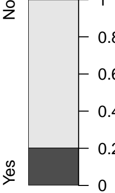
Node 3 (n = 1667)
