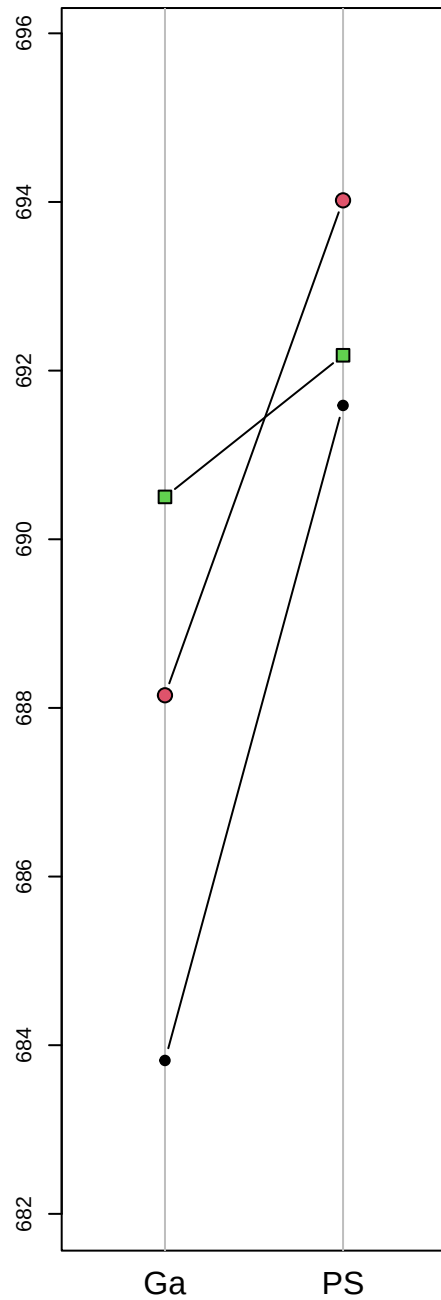
BIC
