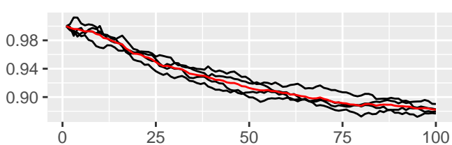
nu
