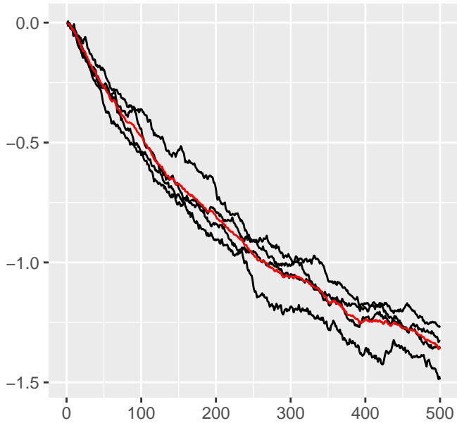
nu
