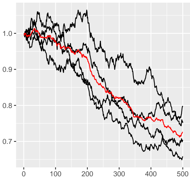
nu
