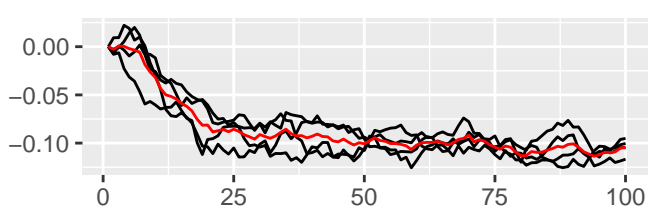
mu
