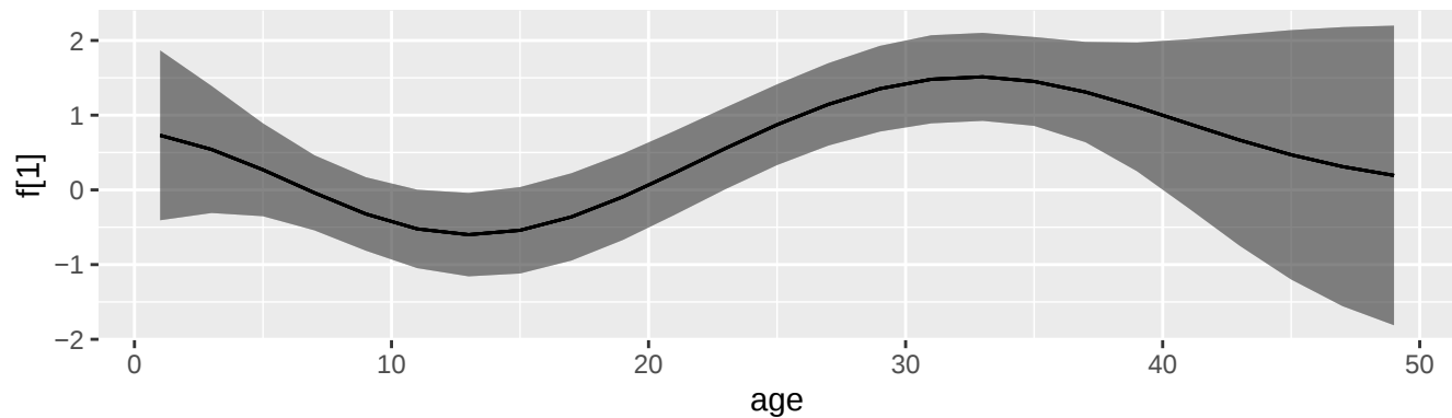
gp_vm(dis_age)
