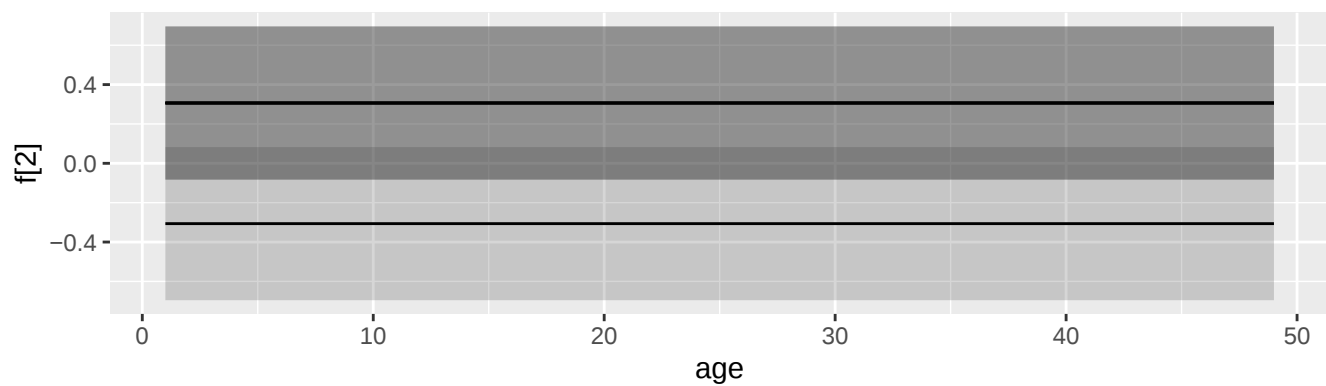
sum
