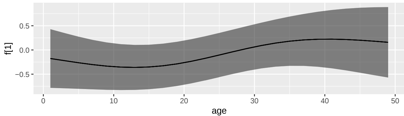
zs(sex)
