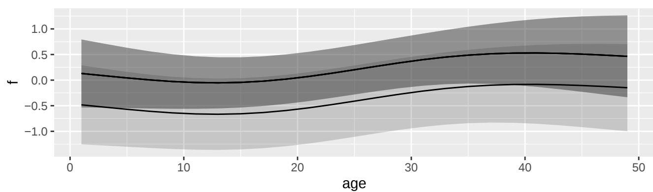
sum
