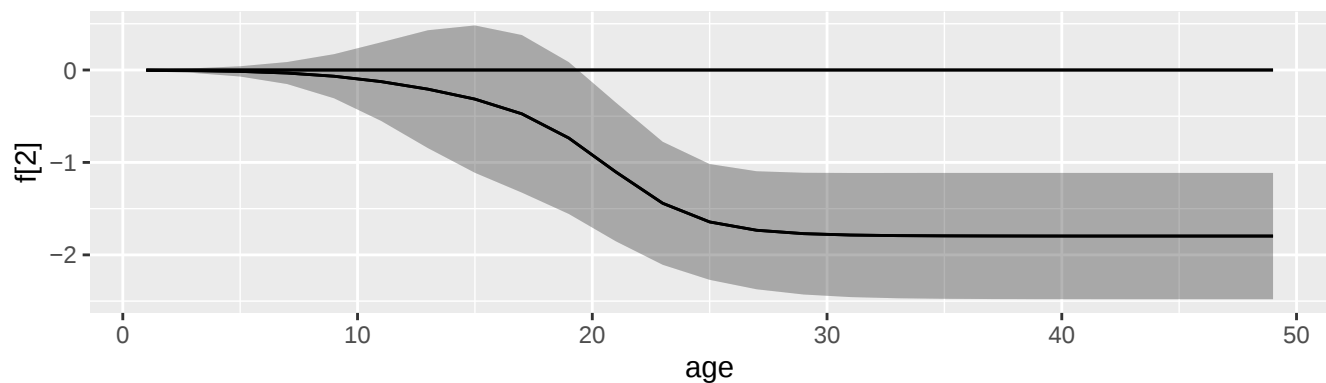
sum
