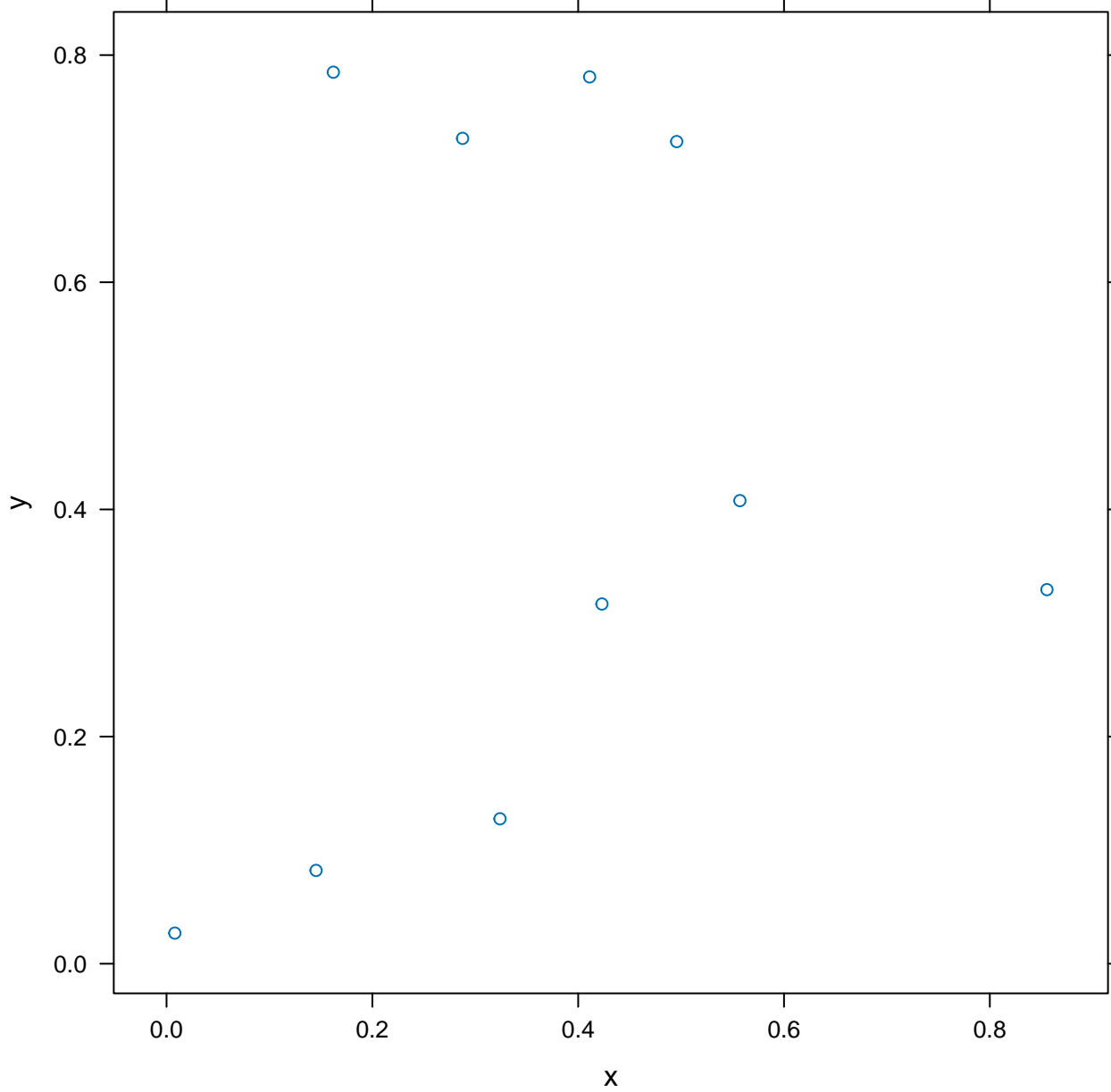
xyplot(y ~ x)
