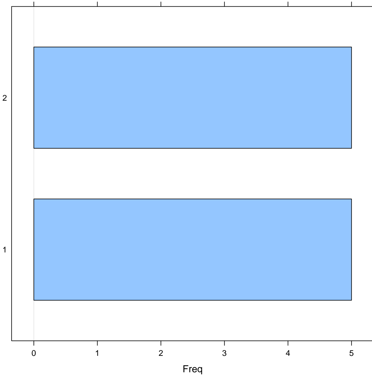
barchart(g2)
