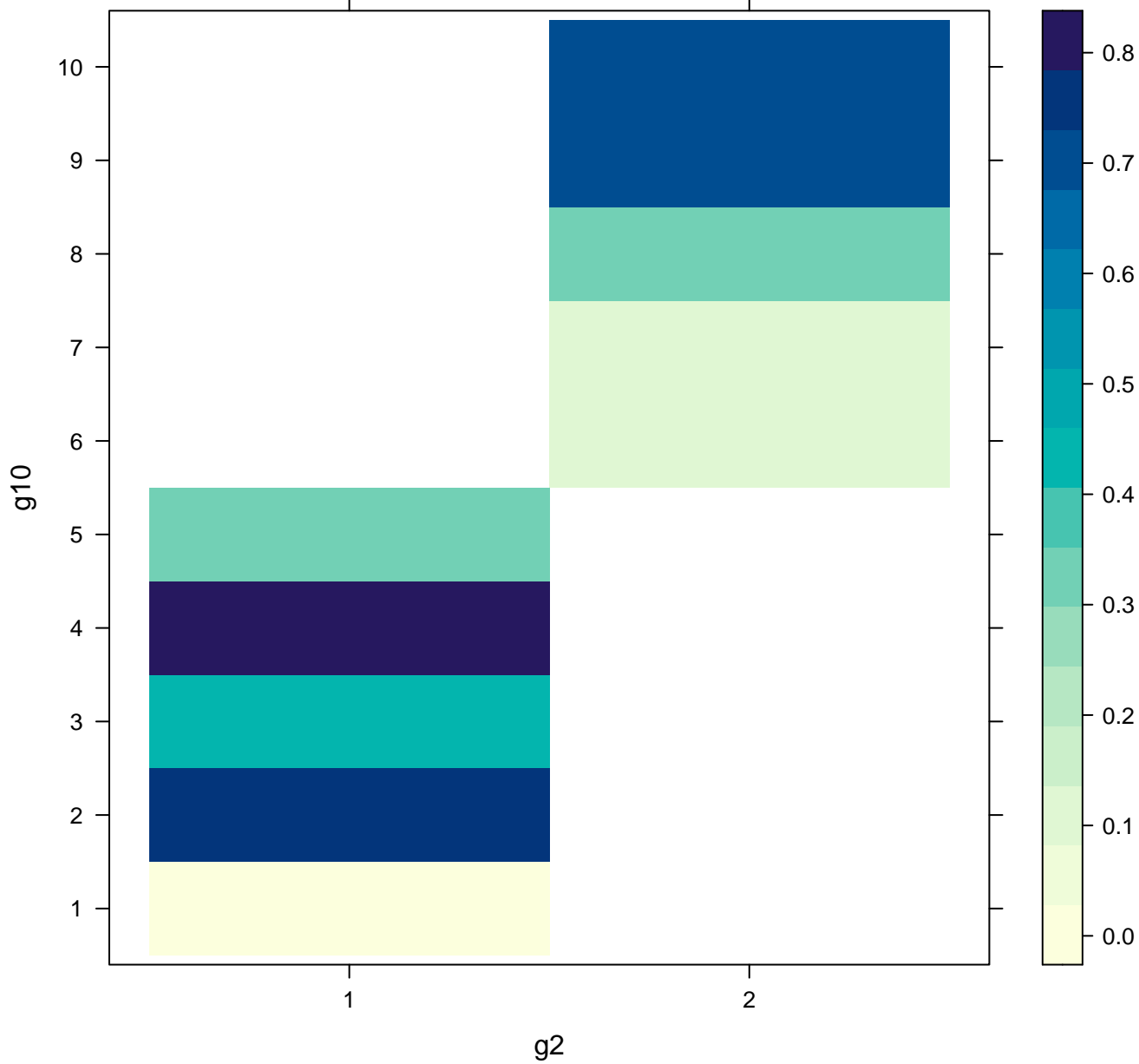
levelplot(y ~ g2 + g10)
