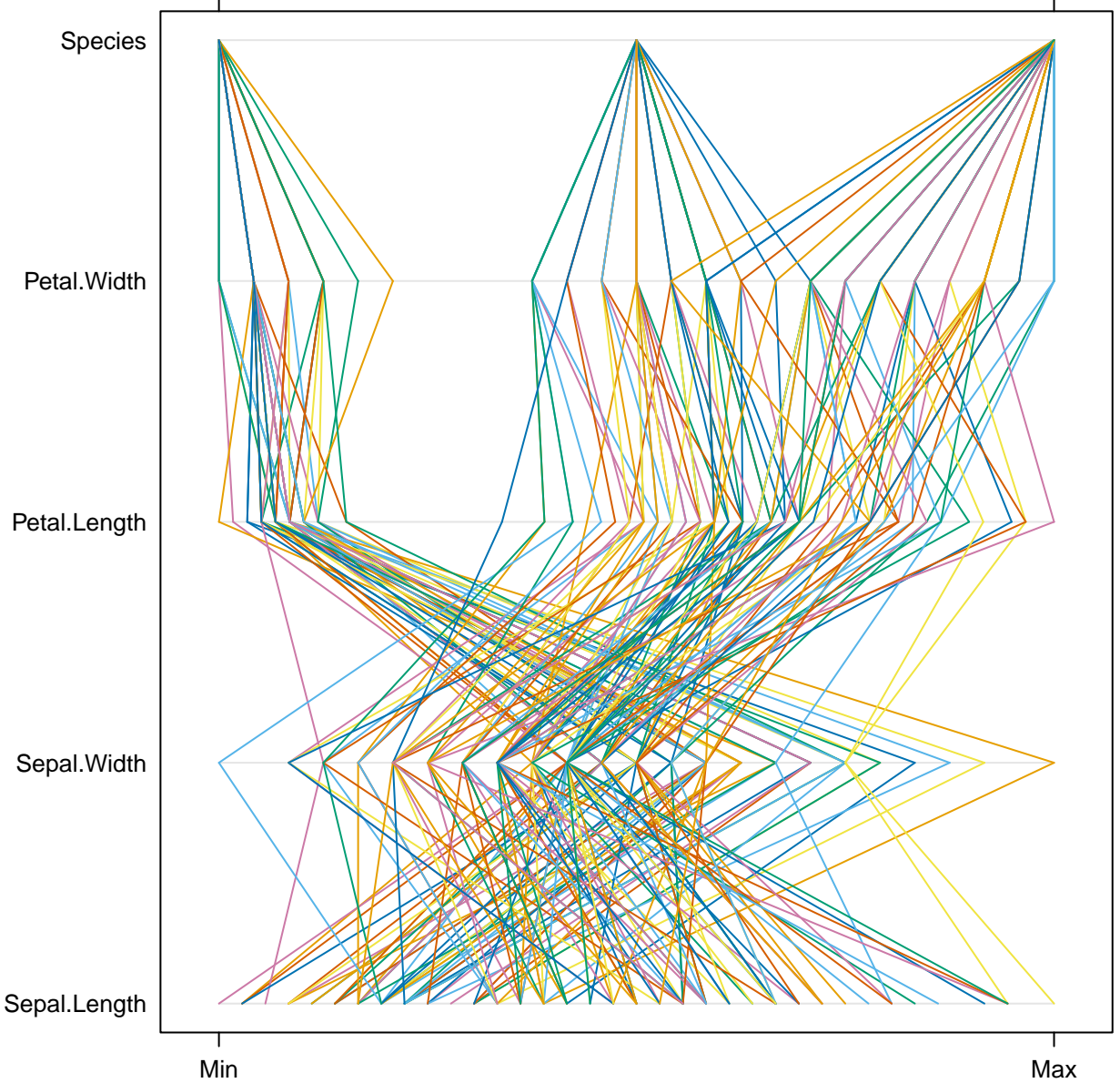
parallelplot(iris)
