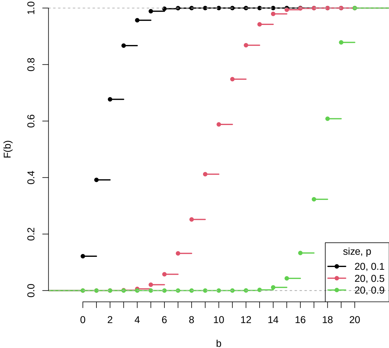
Binomial (size, p) c.d.f.
