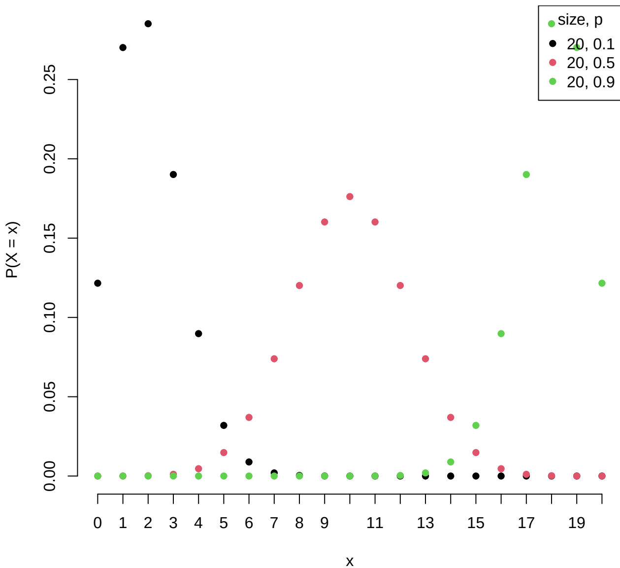
Binomial (size, p) p.m.f.
