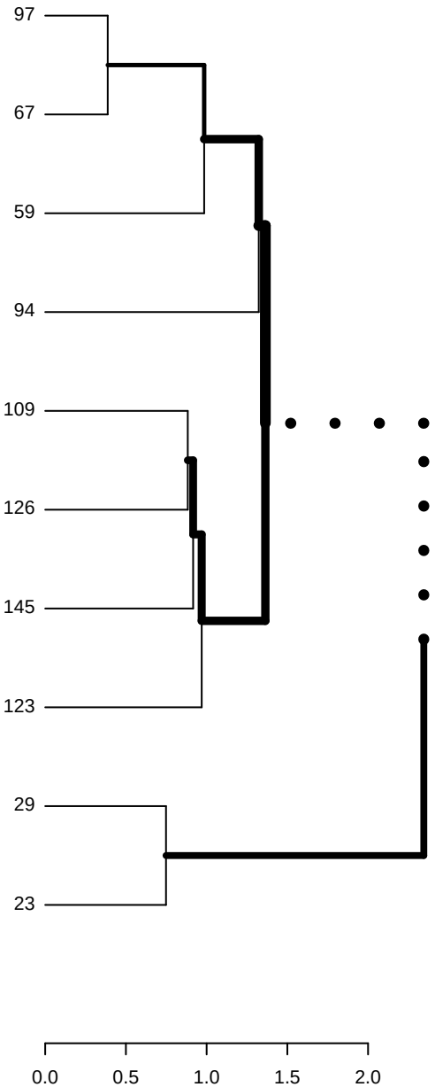
dendrogram2
