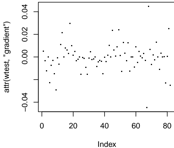
Gradient
