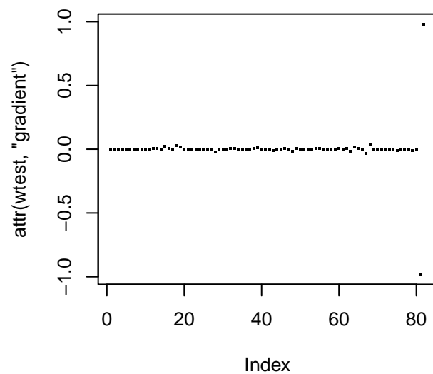
Gradient
