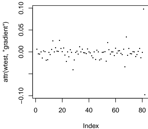
Gradient
