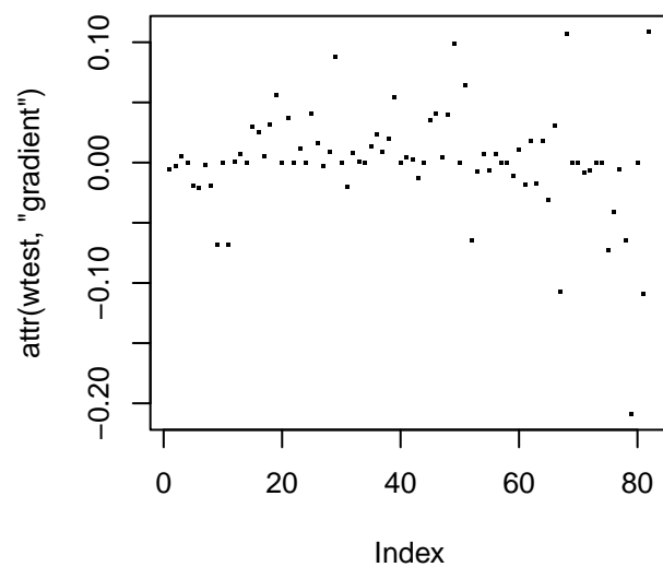
Gradient
