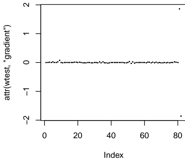
Gradient
