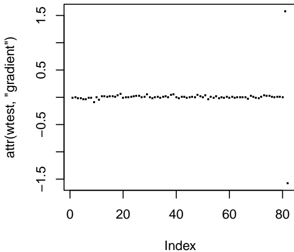
Gradient
