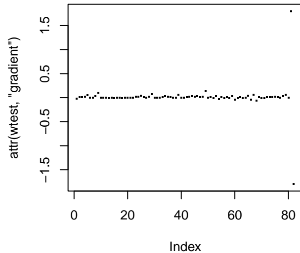
Gradient
