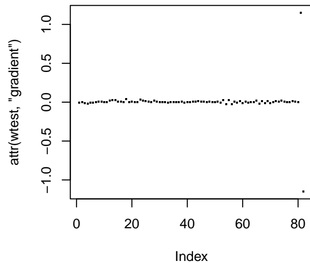
Gradient
