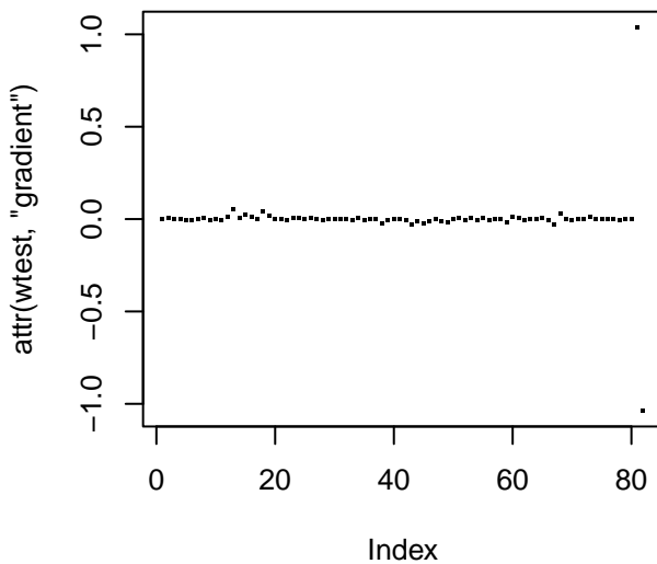
Gradient
