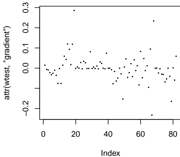
Gradient
