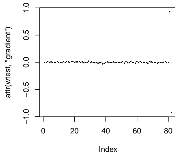
Gradient
