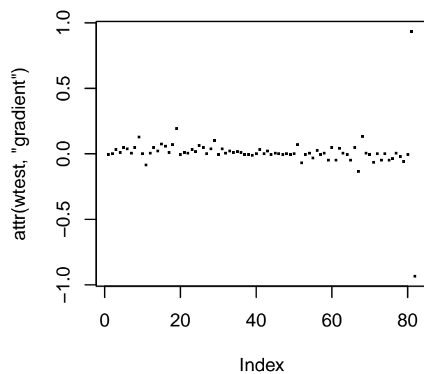
Gradient
