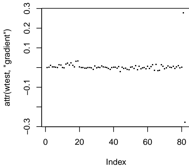
Gradient
