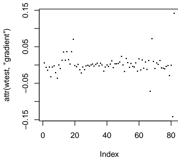
Gradient
