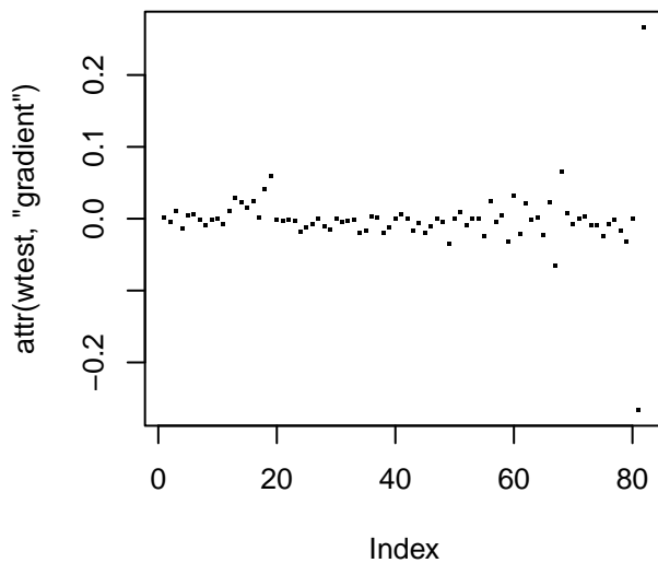
Gradient
