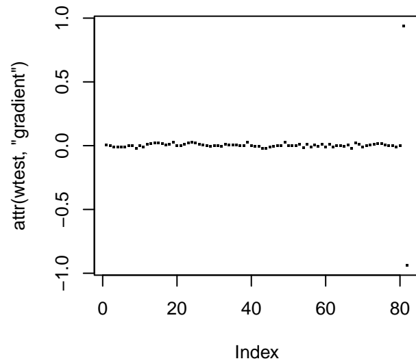
Gradient
