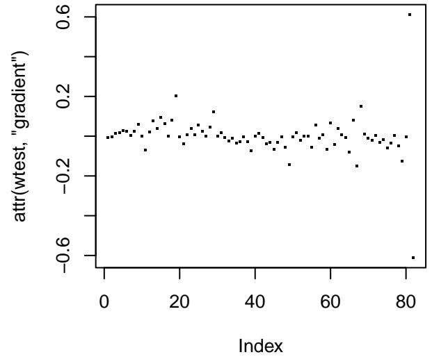
Gradient
