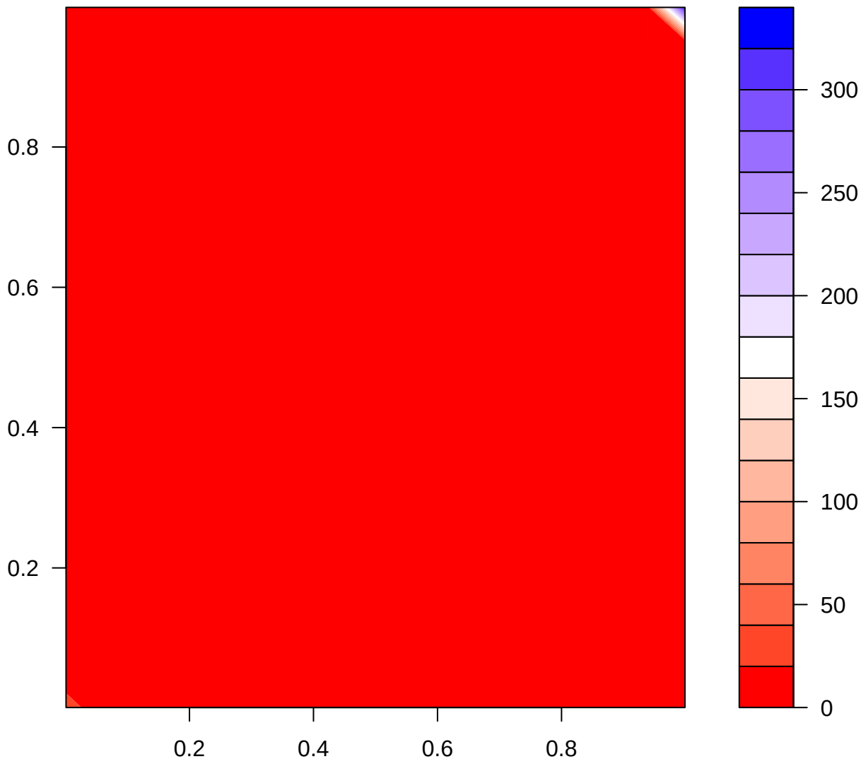
Density( galambosCopula(1.285) )
