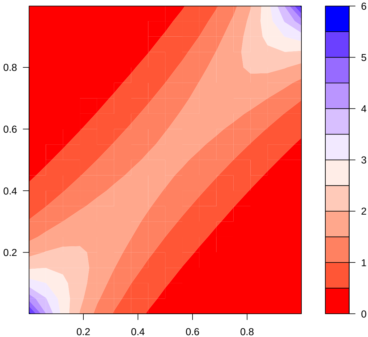
Density( frankCopula(5.736) )
