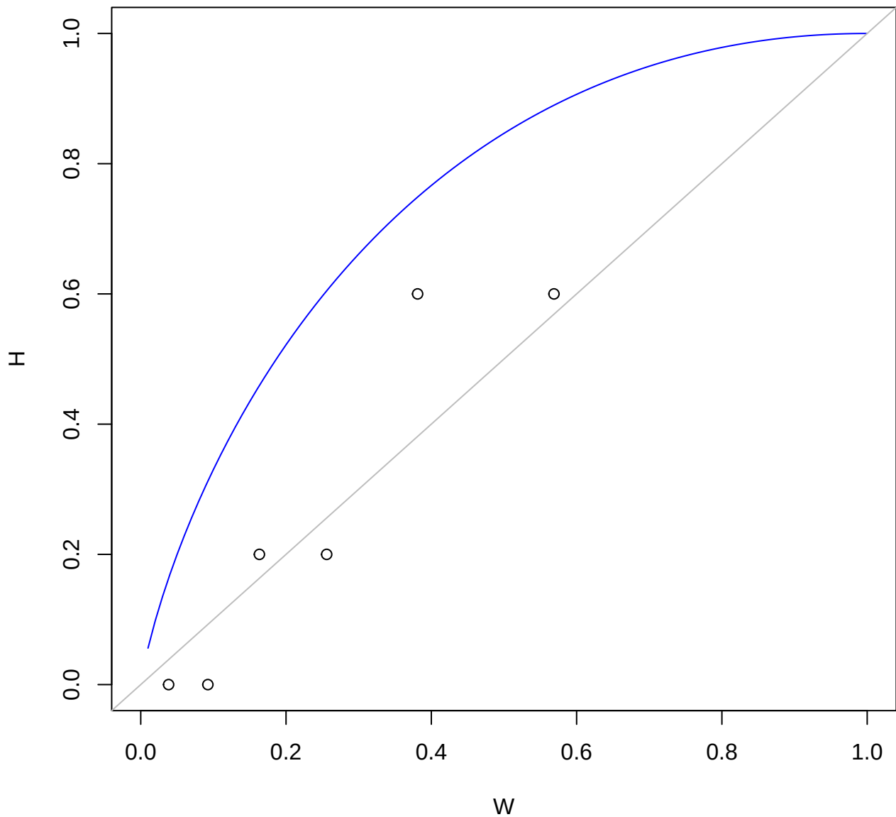
Kplot(X)
