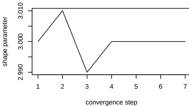
GEV parameter values being tested
