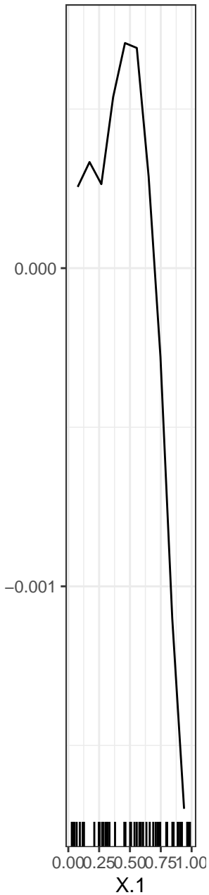
X.1 ... NA
