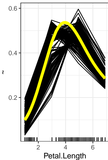
PDP – versicolor
