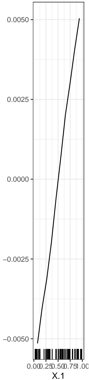
X.1 ... NA
