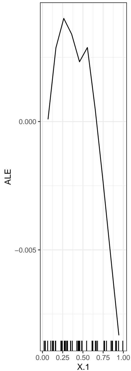
X.1 ... Y.3
