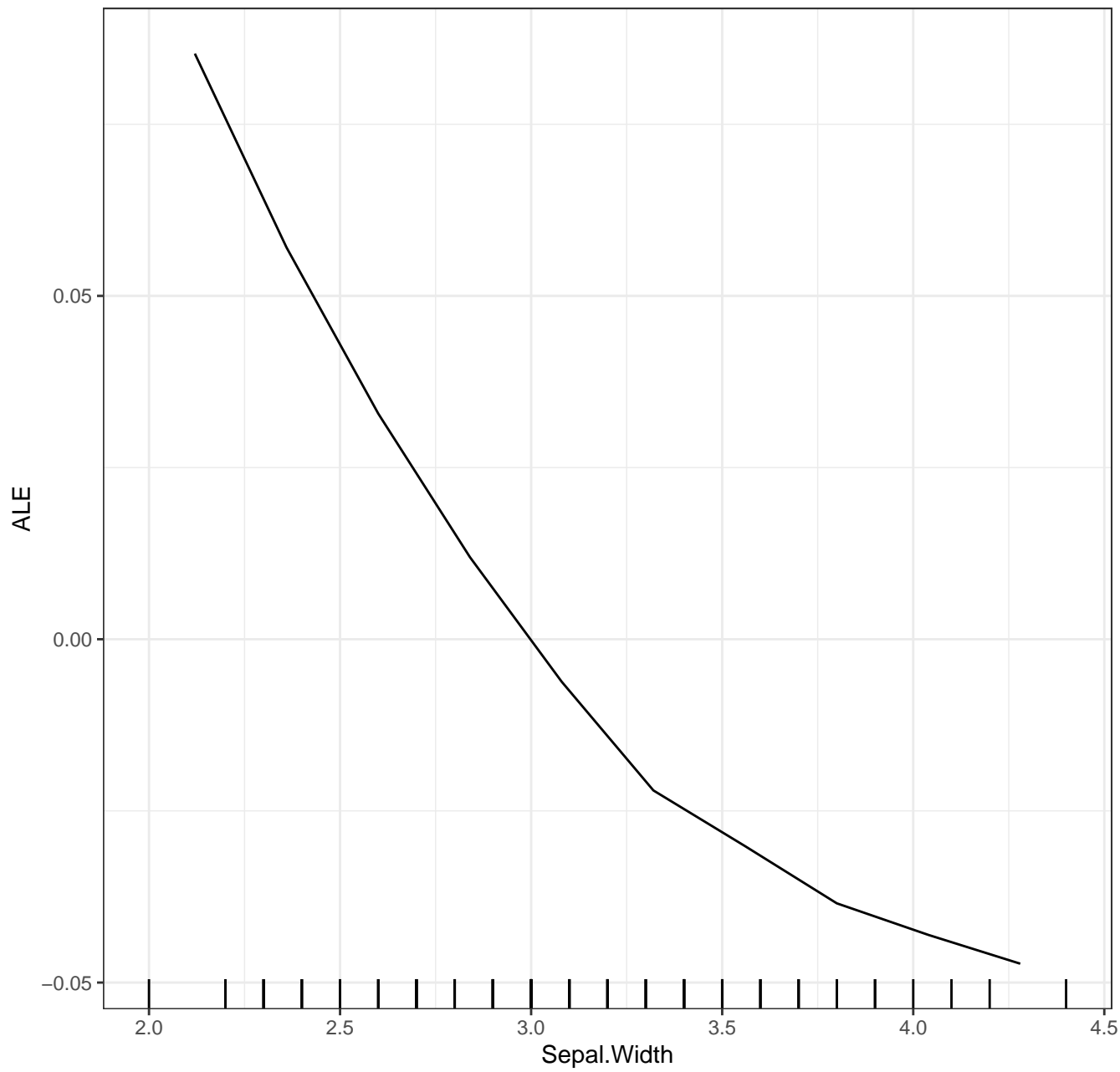
Sepal.Width ... Species
