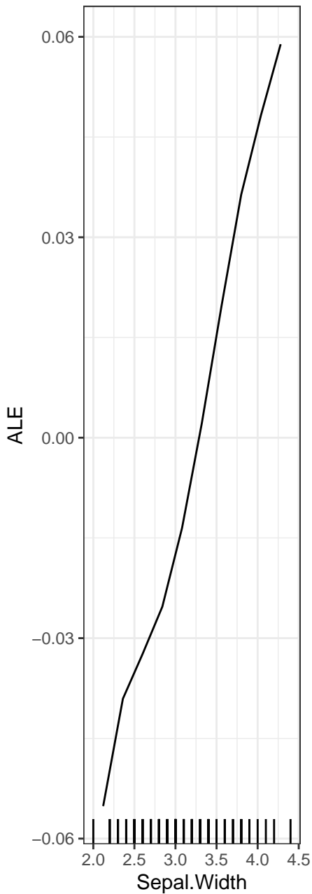
Sepal.Width ... setosa:
