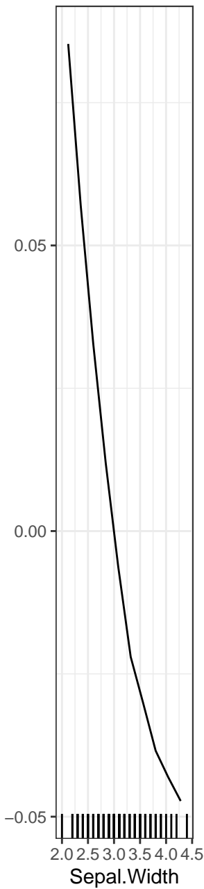
Sepal.Width ...
