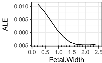
Petal.Width ... setos:
