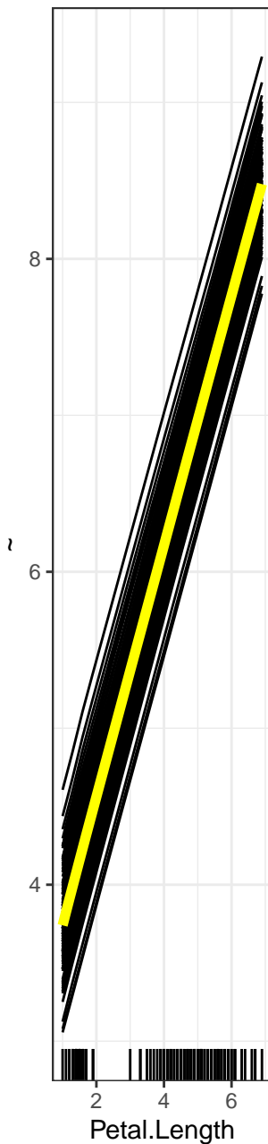
PDP
