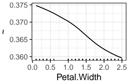
PDP – versicolor
