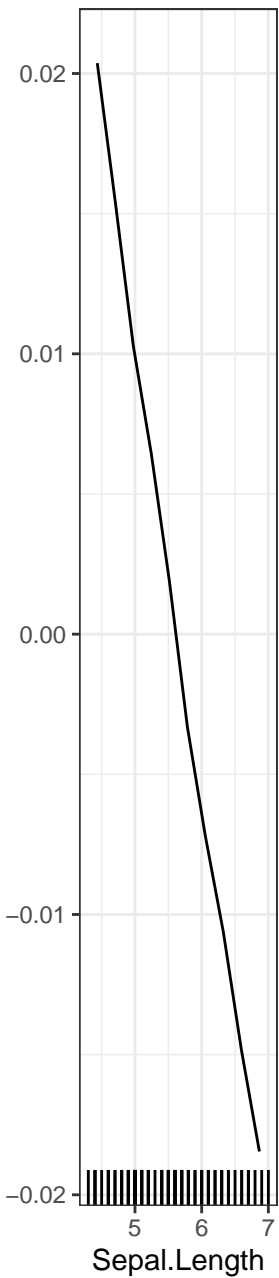
Sepal.Length
