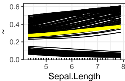
PDP – versicolor
