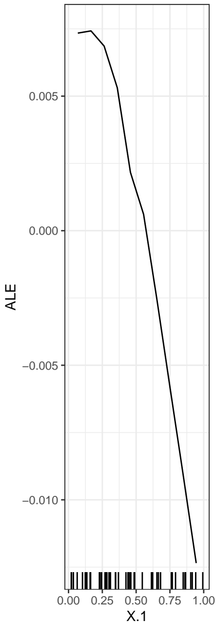
X.1 ... Y.1
