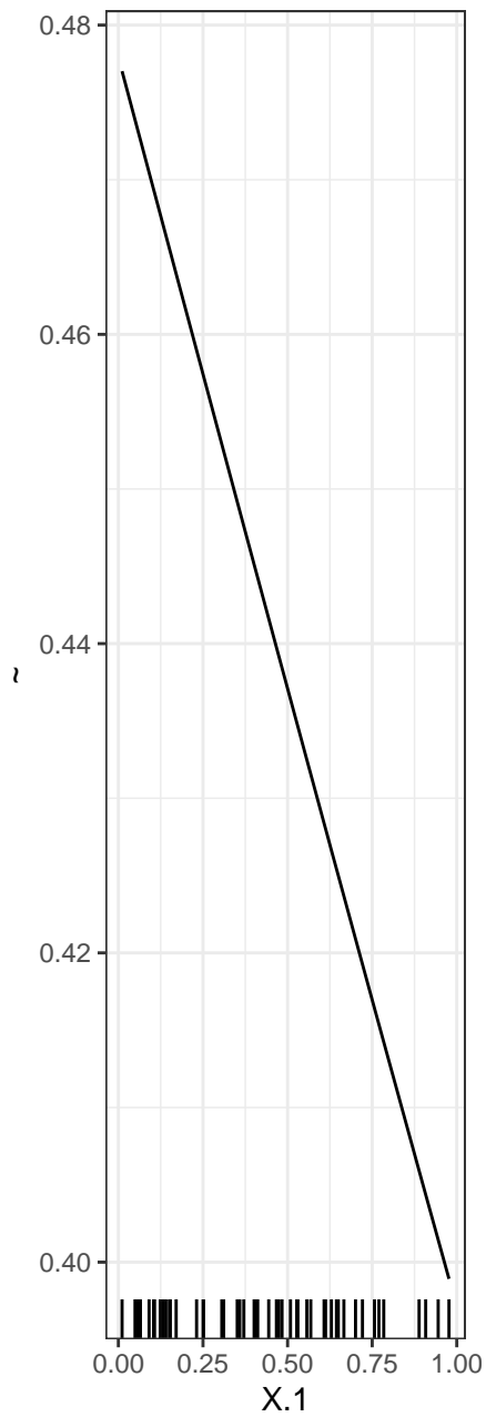
PDP
