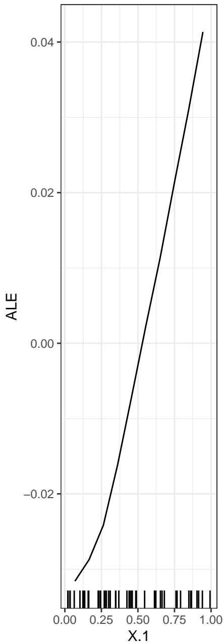
X.1 ... Y.2
