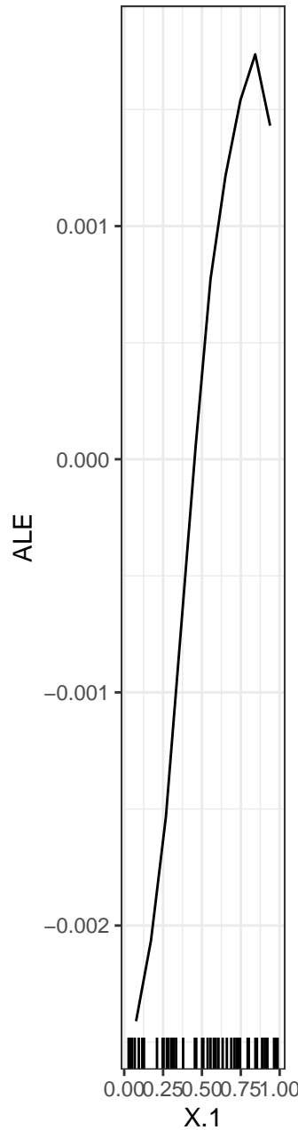
X.1 ... NA
