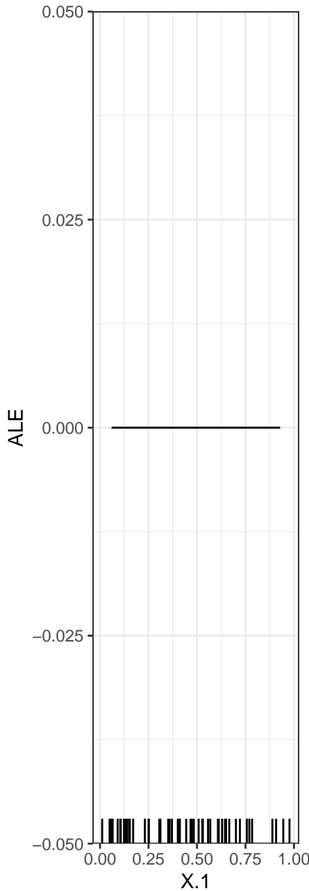
X.1 ... Y.3
