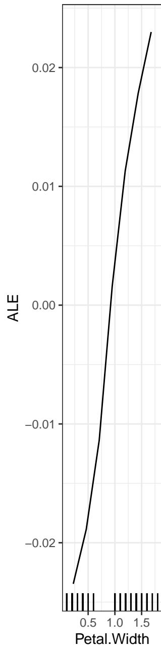
Petal.Width ...
