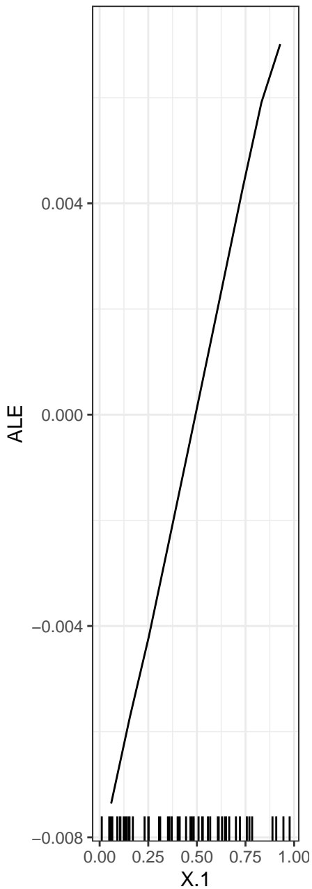
X.1 ... Y.1
