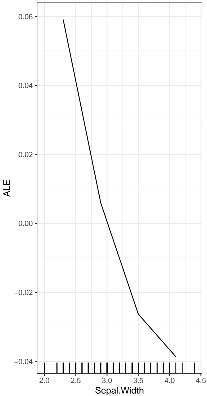
Sepal.Width ... Species
