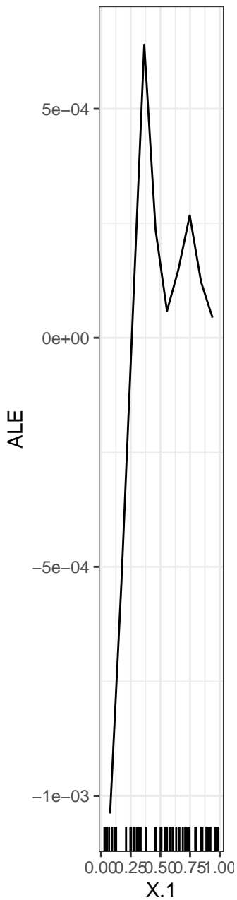
X.1 ... NA
