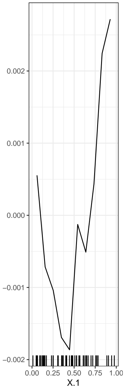
X.1 ... Y.1
