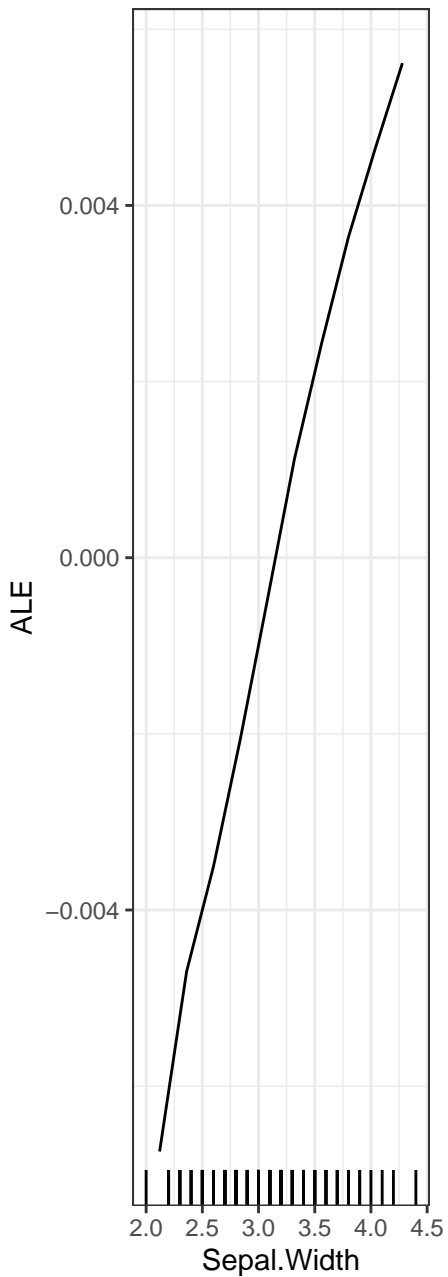
Sepal.Width ... setos
