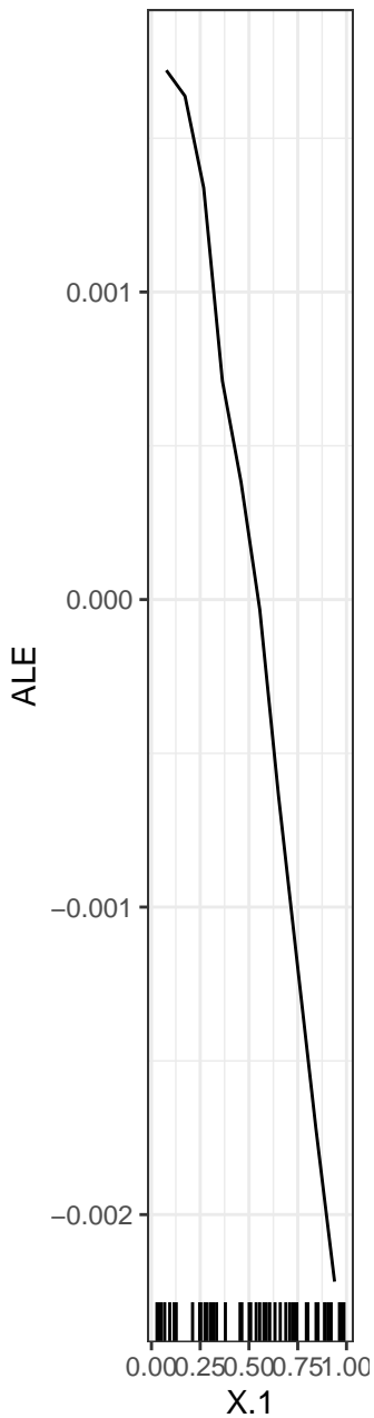
X.1 ... Y
