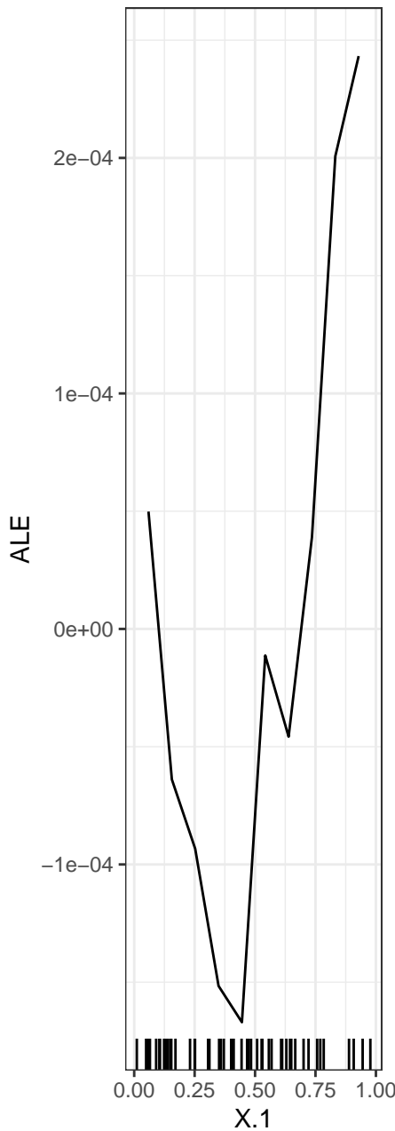
X.1 ... Y.3
