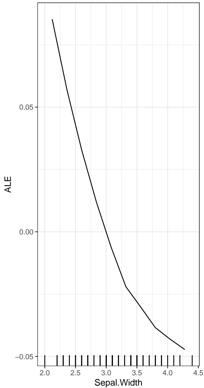
Sepal.Width ... Species
