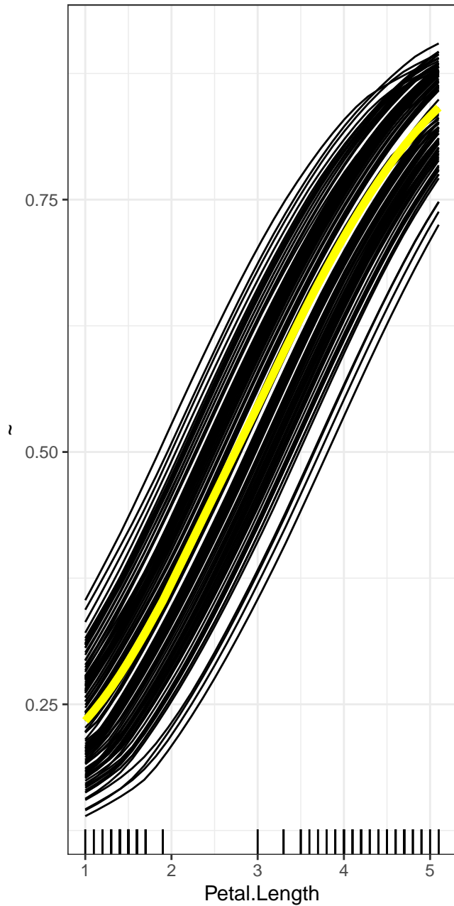
PDP
