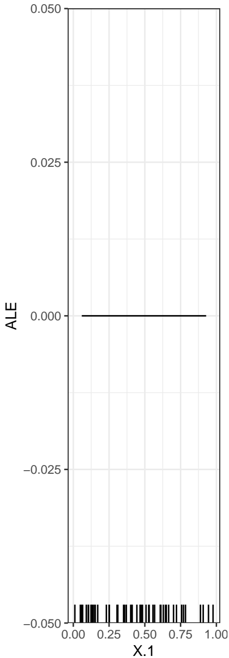
X.1 ... Y.2
