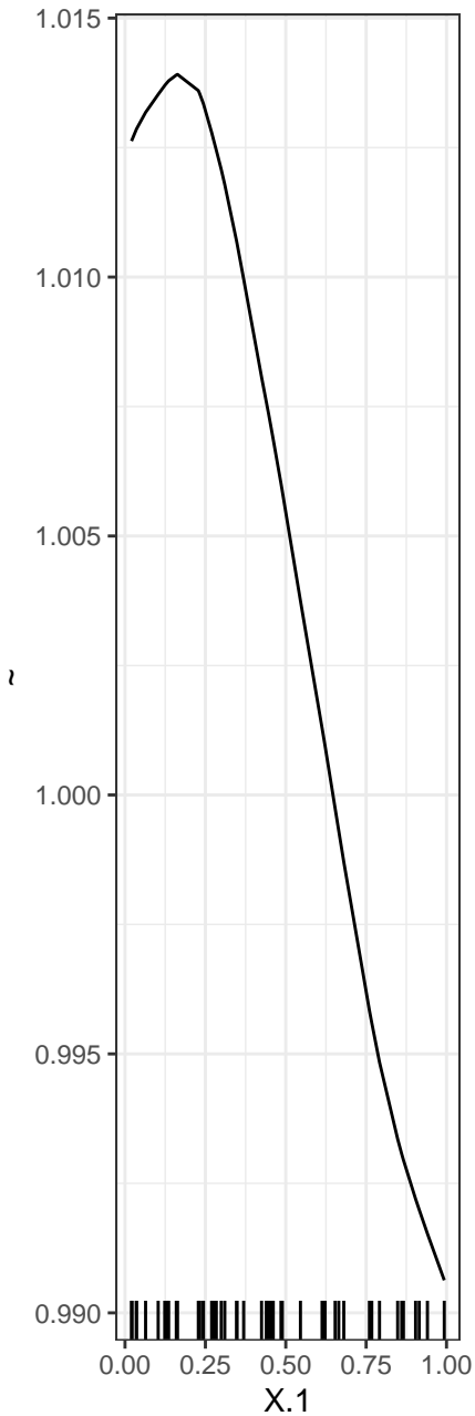
PDP
