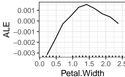
Petal.Width ... versic
