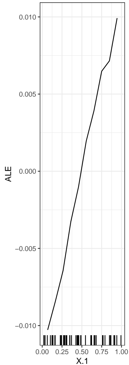
X.1 ... Y.3
