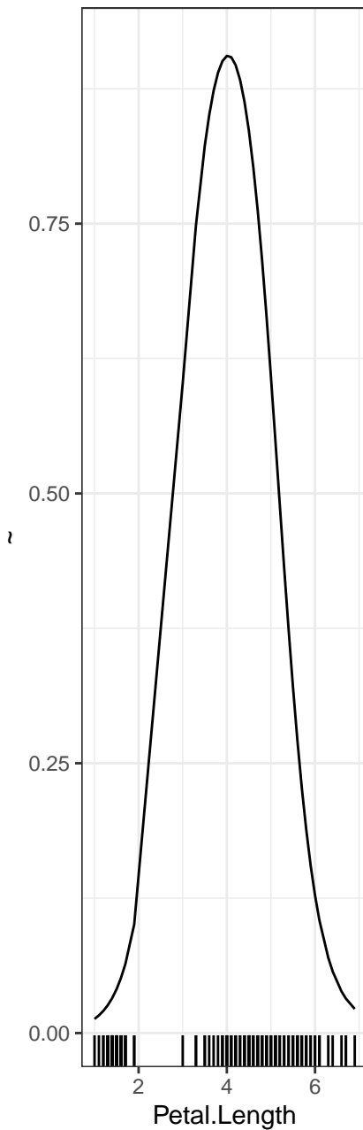
PDP – versicolor
