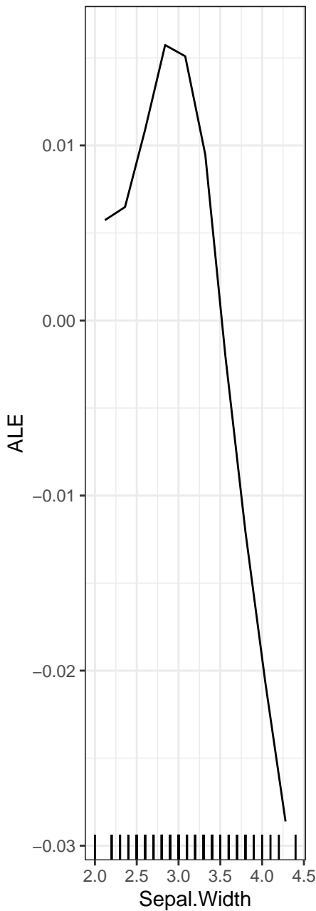
Sepal.Width ... versicol:
