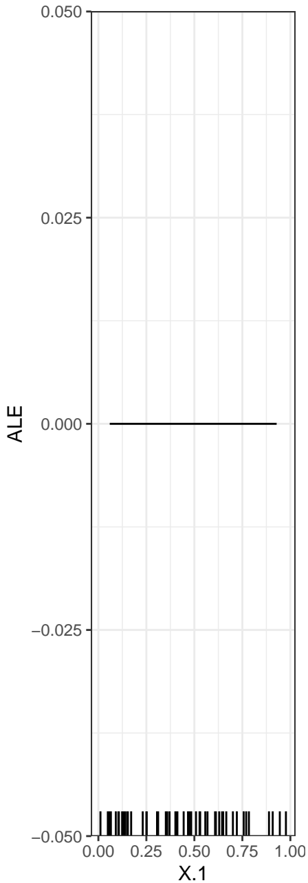
X.1 ... Y.1
