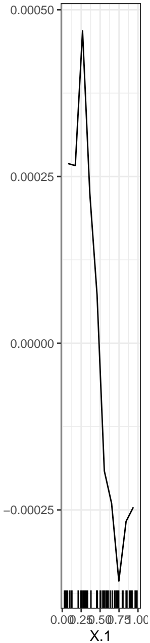
X.1 ... Y
