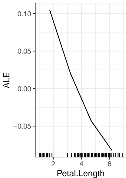
Petal.Length ... setos
