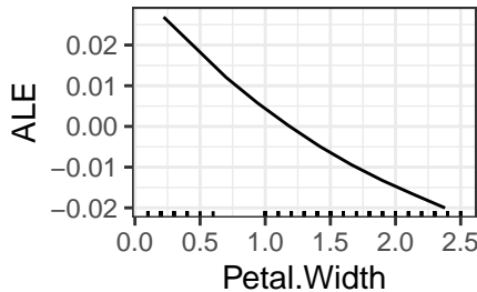
Petal.Width ... setosa
