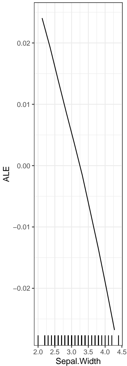
Sepal.Width ... versic
