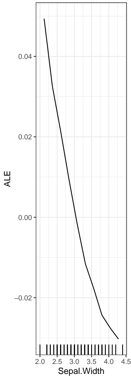
Sepal.Width ... virginica:
