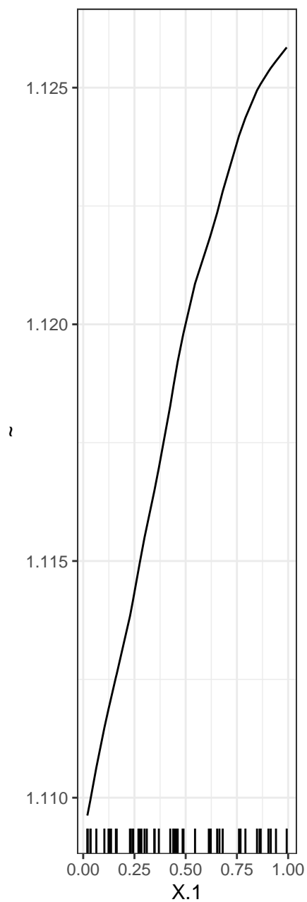
PDP
