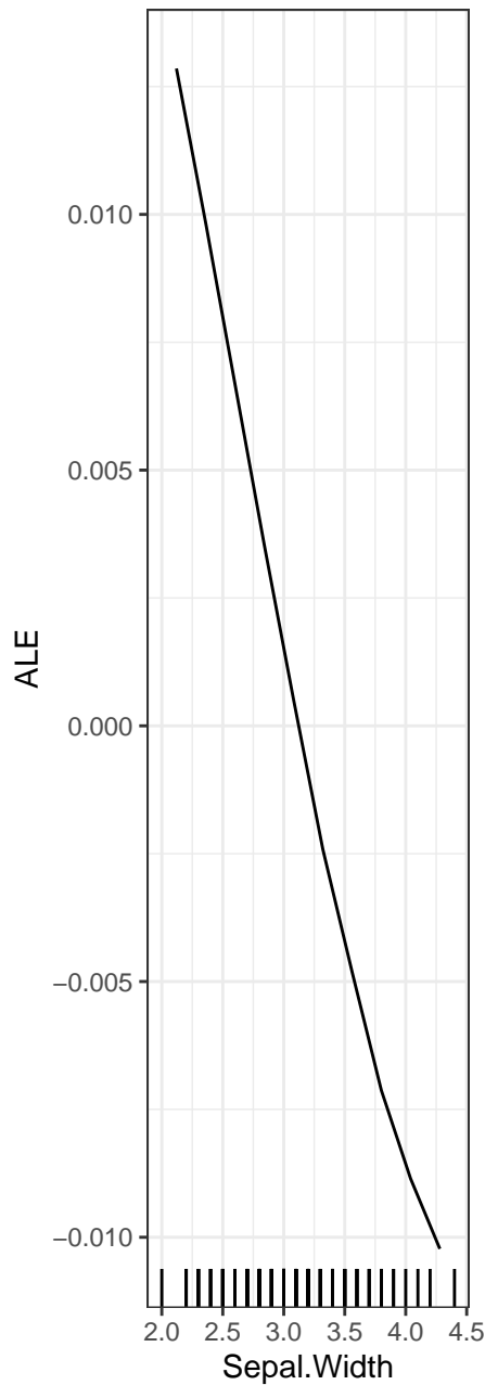
Sepal.Width ... virgin
