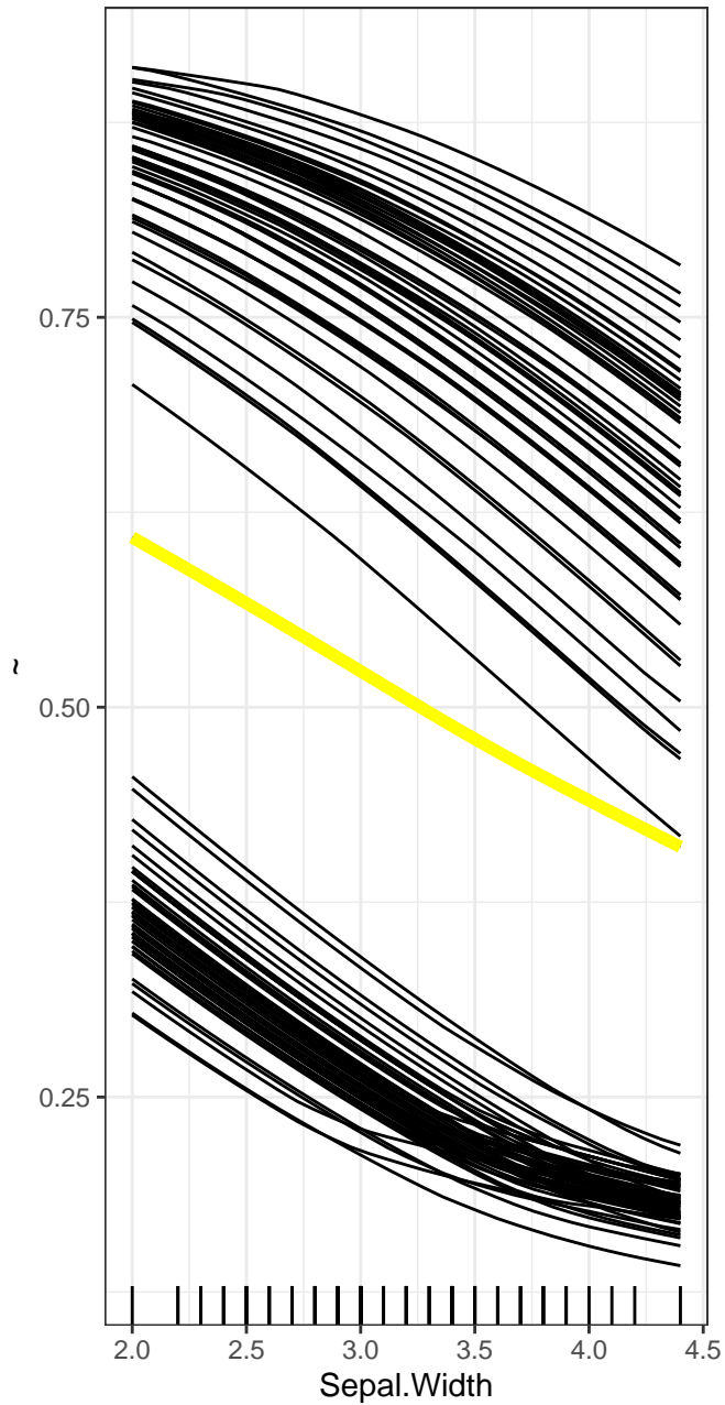
PDP
