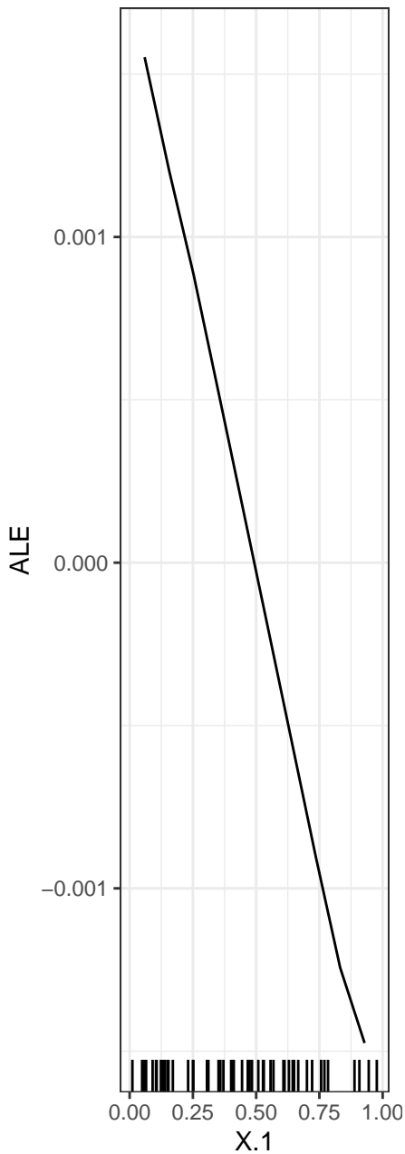
X.1 ... Y.2
