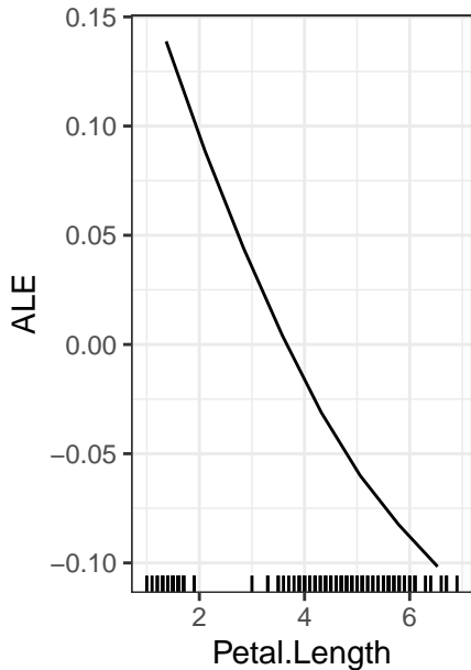
Petal.Length ... setos
