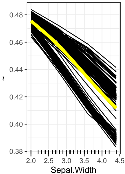
PDP – versicolor
