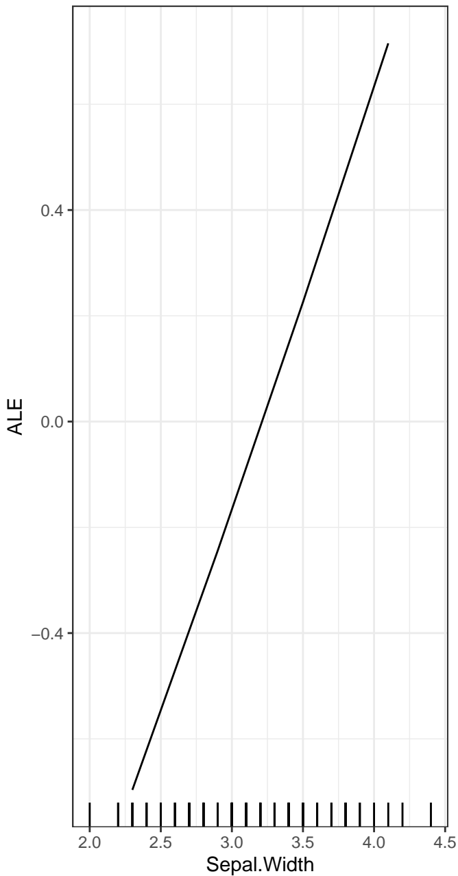
Sepal.Width ... Sepal.Length
