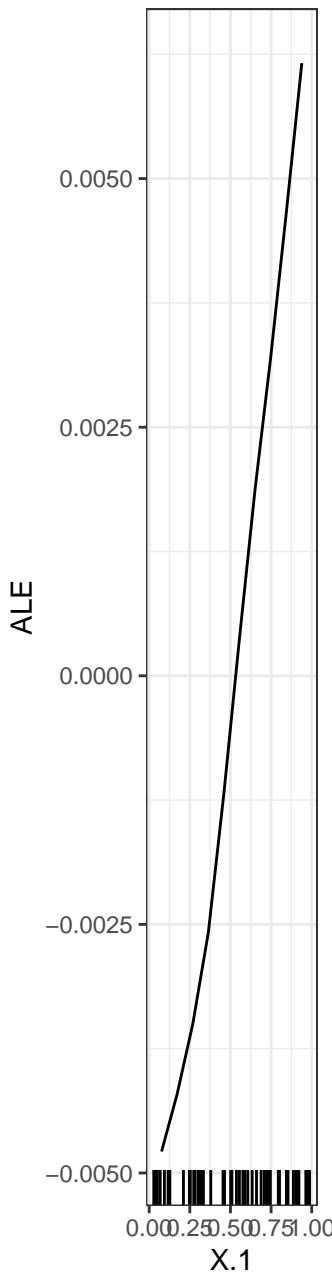
X.1 ... NA
