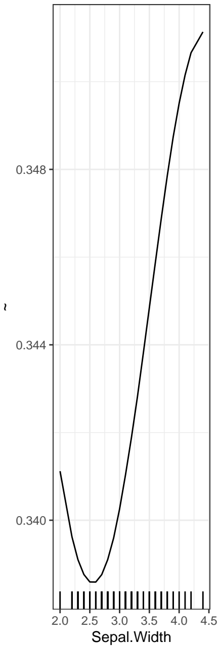
PDP – versicolor
