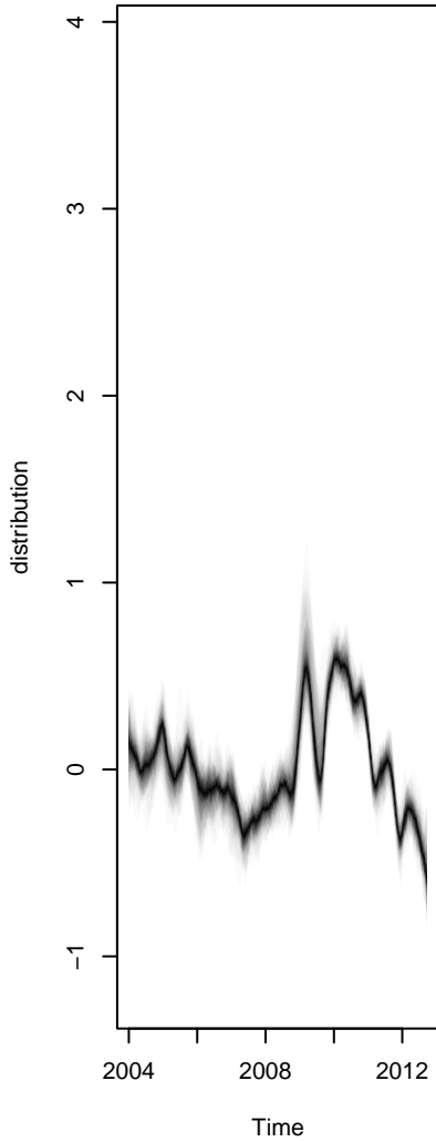
trend
