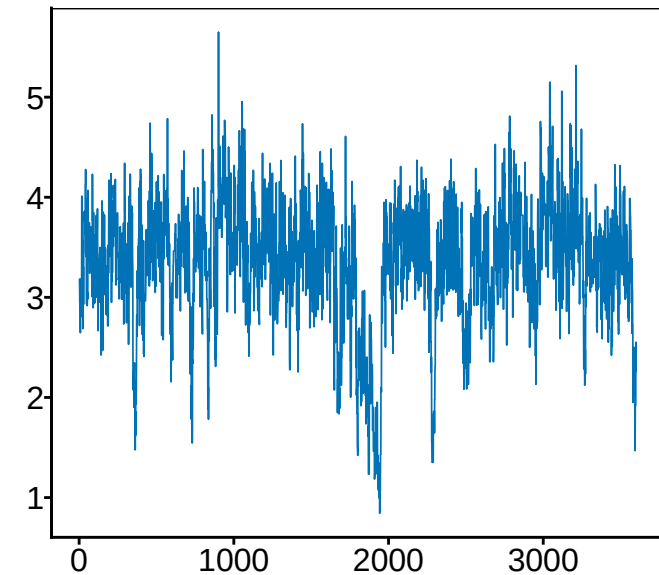
Chain nr 3
