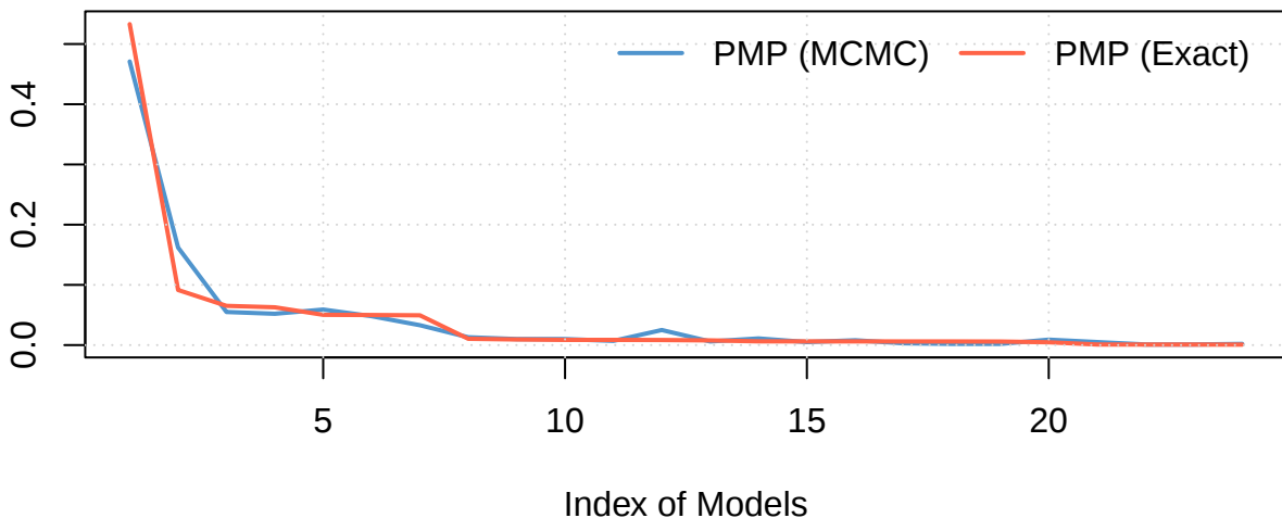
Posterior Model Probabilities (Corr: 0.9845)
