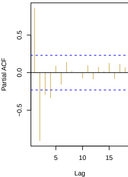
PACF
