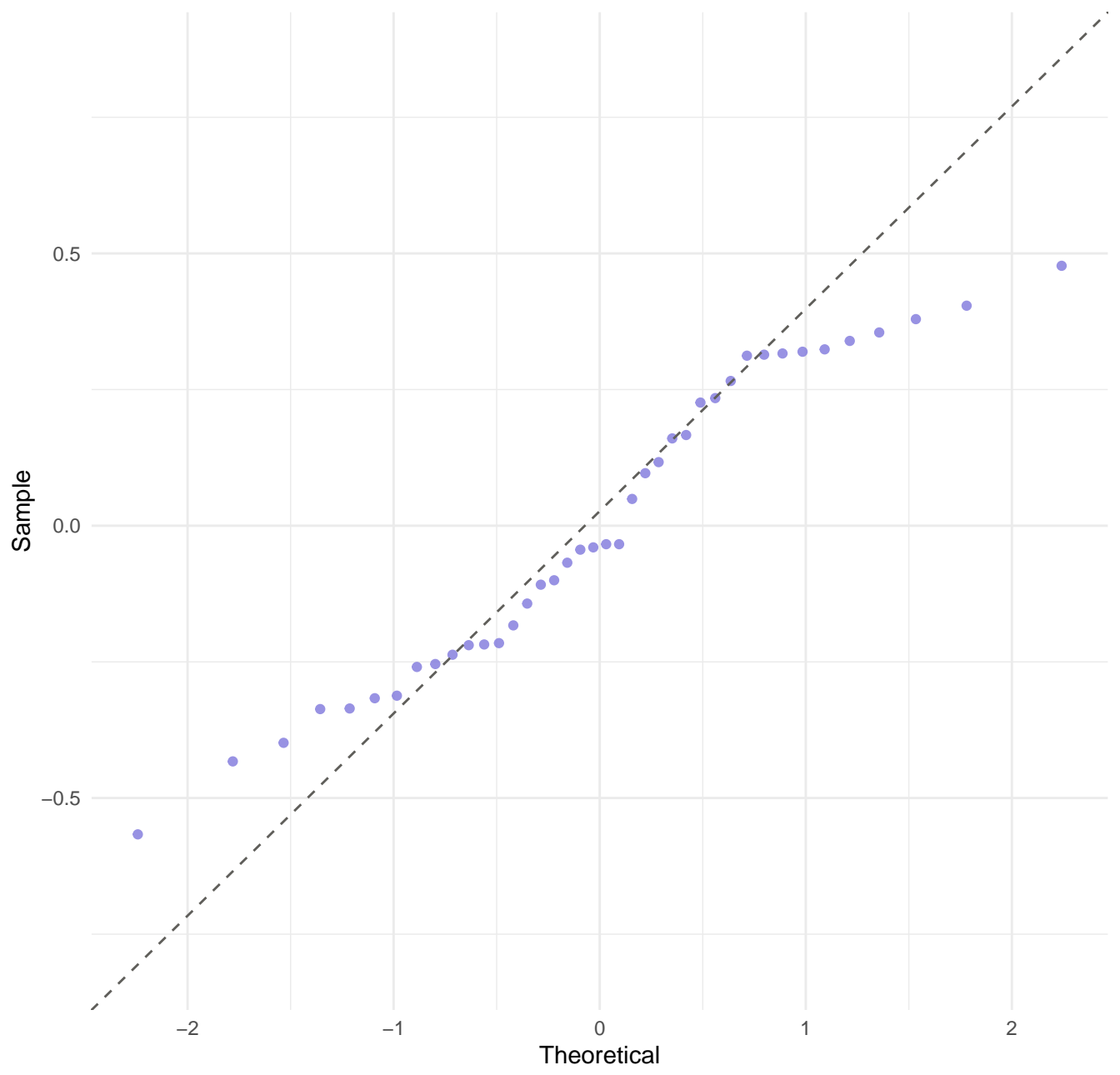
Normal Q-Q
