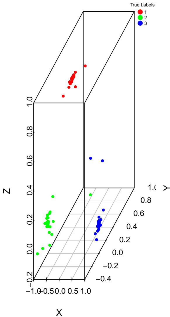
True Labels
