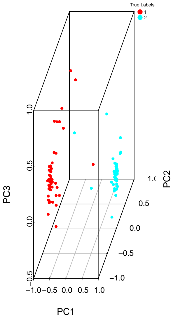
True Labels
