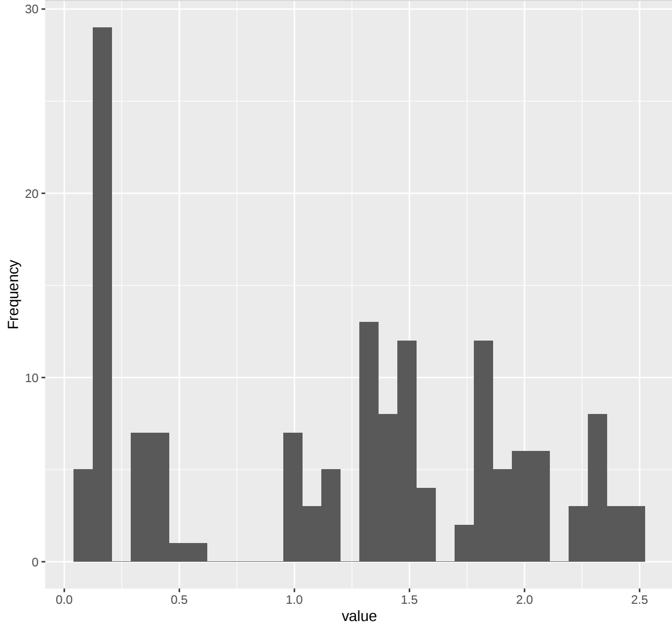
Petal.Width
